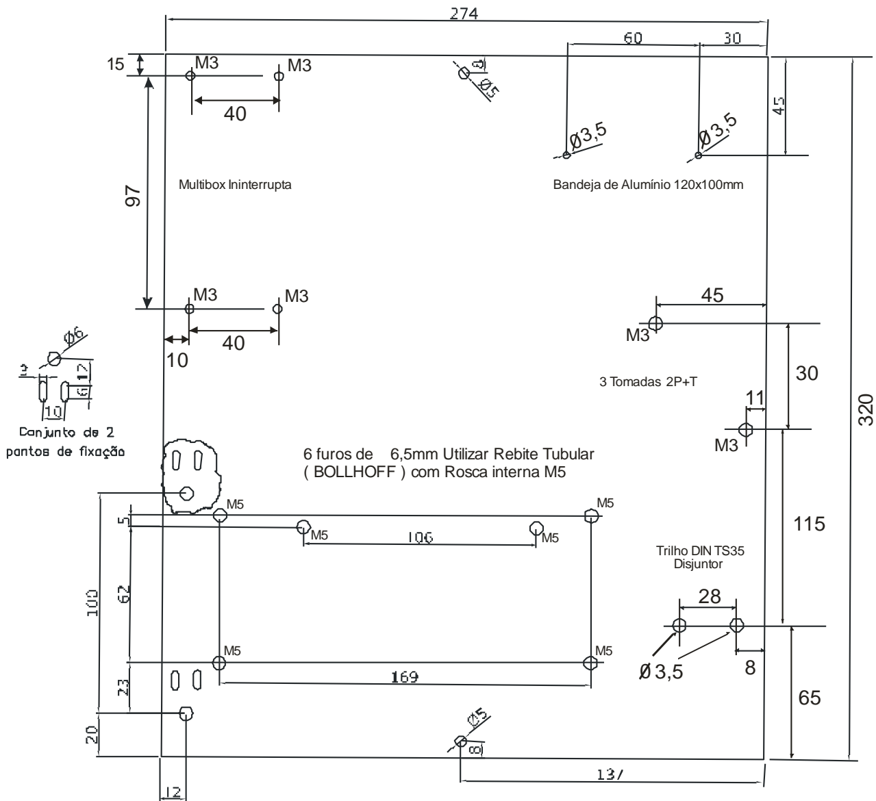
Chapa 1,5mm com Pintura Eletrostática Laranja RAL2004
